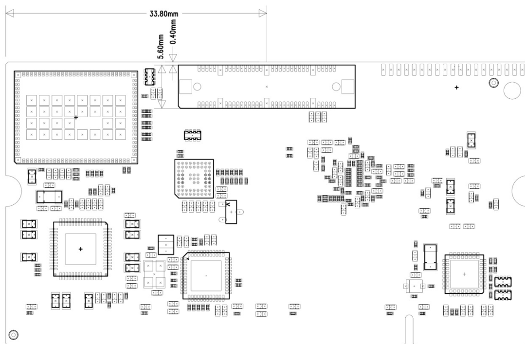
Dimensions (mm) of the Trizeps VIII Mini module (bottom view)
