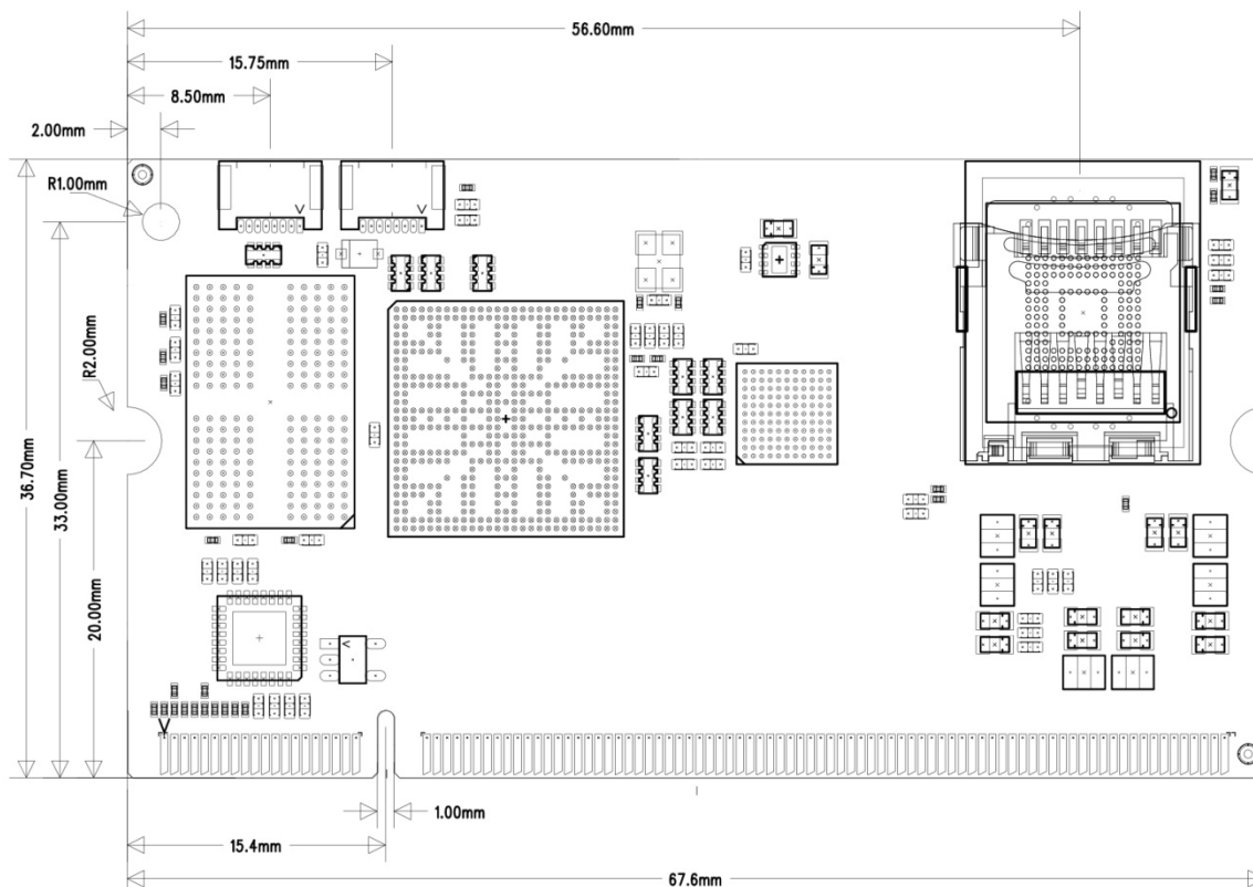
Dimensions (mm) of the Trizeps VIII Mini module (top view)
